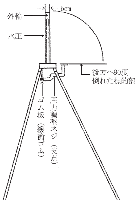
側 面（標的部が倒れた図）
