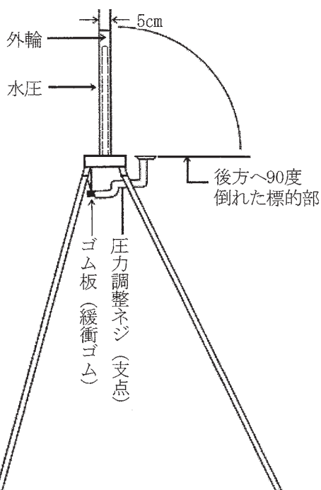
側 面（標的部が倒れた図）
